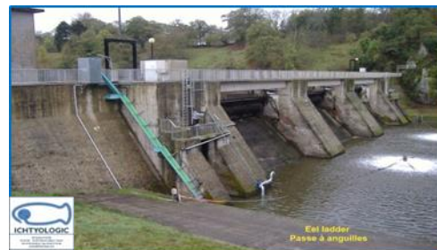
Barrage d'Apremont, Vie \Delta h = 11.50 m
